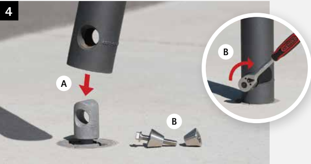
A) Poller auf Verbindungsstück setzen B) Spannkegelsatz einsetzen und festziehen
