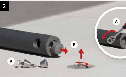
A) Spannkegelsatz im Poller lösen und herausnehmen B) Gebrochene Verbindungsstücke aus Poller und Bodenhülse entnehmen
